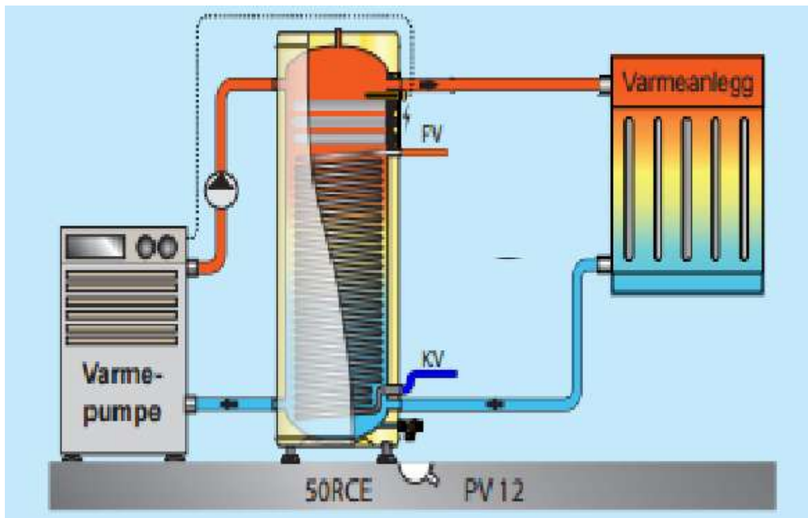
Standard oppsett med akkumulatortank m/elkolber og spiral til forvarming av VV.
